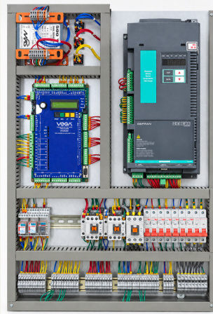
VEGA 200 / GEFAN
